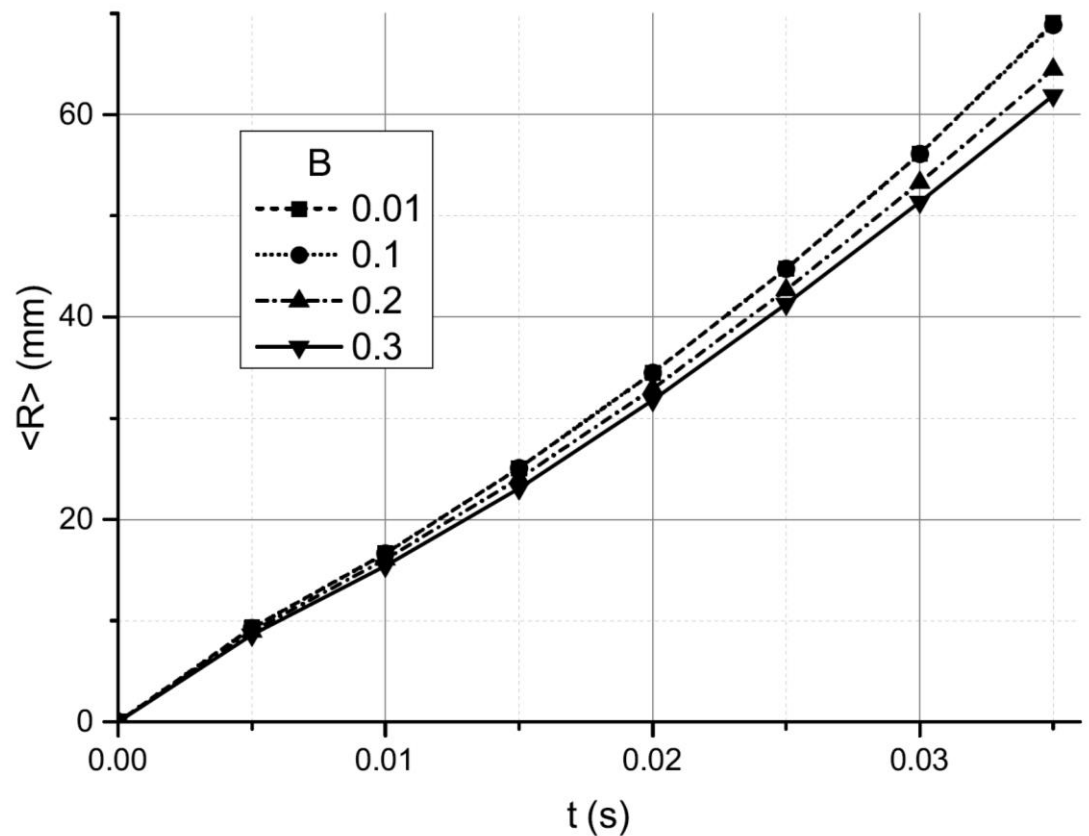
График зависимости среднего радиуса фронта пламени от времени при различных пороговых коэффициентах бинаризации 0.01, 0,1, 0,2 и 0,3
