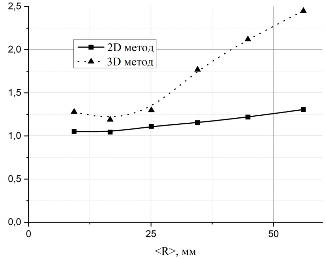
График зависимости коэффициента складчатости от радиуса фронта пламени. Водородно-воздушная смесь с 15% содержанием водорода.
