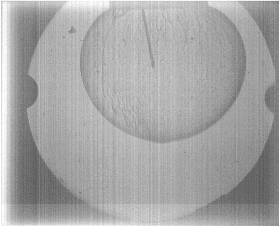
Гладкий фронт богатого пламени
