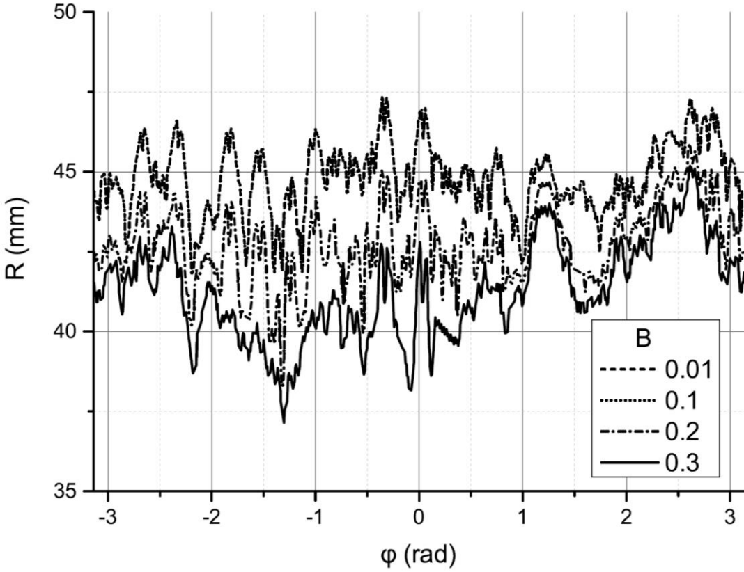
График угловой развертки фронта пламени при разных пороговых значениях бинаризации 0.01, 0,1, 0,2 и 0,3
